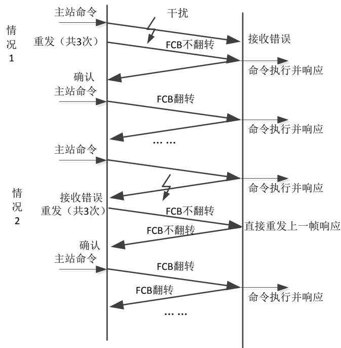
图 43 非平衡链路下的“发送/确认”干扰过程
