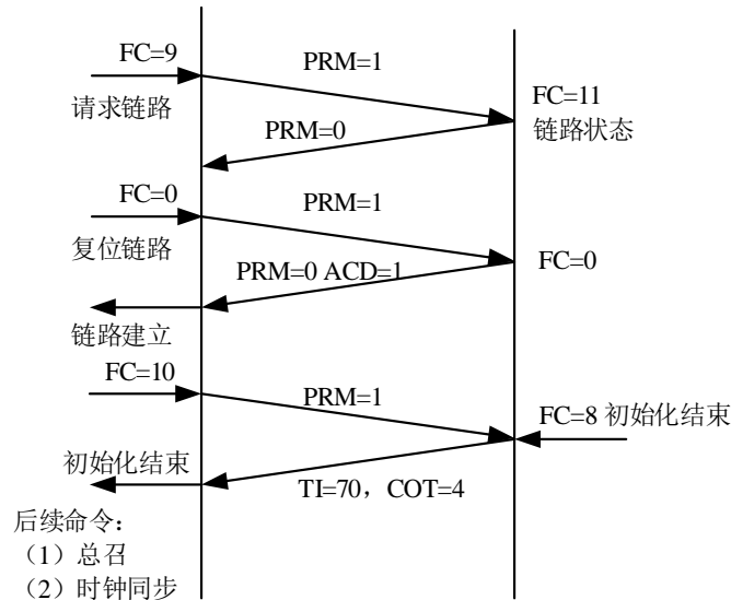
图 2 非平衡链路传输模式中初始化过程
