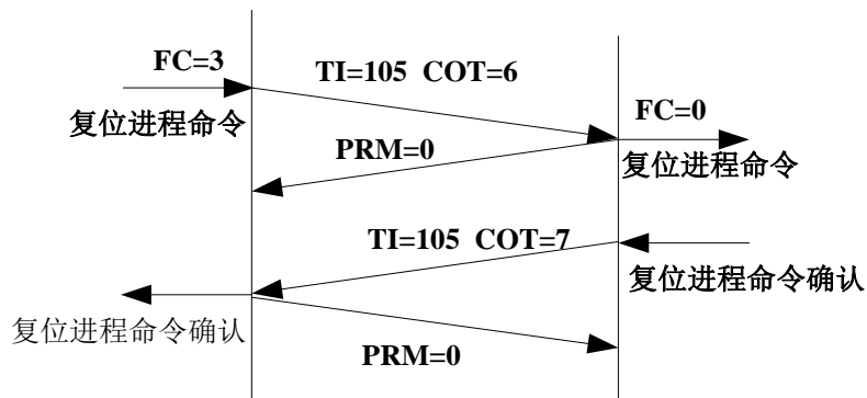
图 20 平衡链路模式下的复位进程过程
