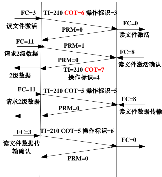
图 23 非平衡传输模式中读文件传输过程
