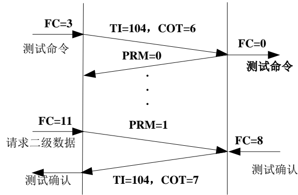
图 14 非平衡链路传输模式中链路测试过程
