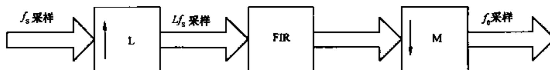
图 B.2 DSP 方案
