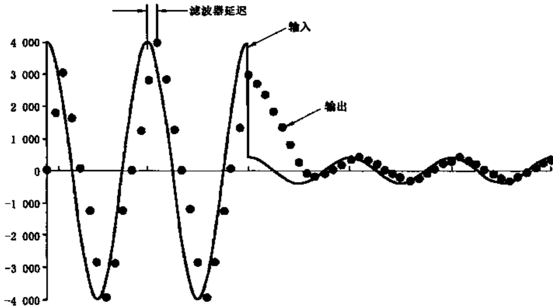
图 B.3 采样率转换实例
